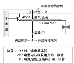
输入输出电路图
